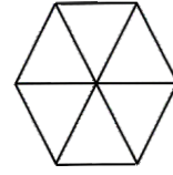
षट्कोन
